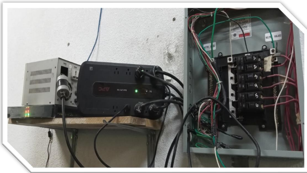
Conexión de UPS provisional para pinspotter
